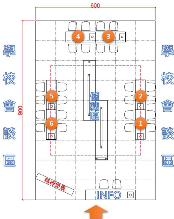
臺灣參展學校會談桌平面配置圖
