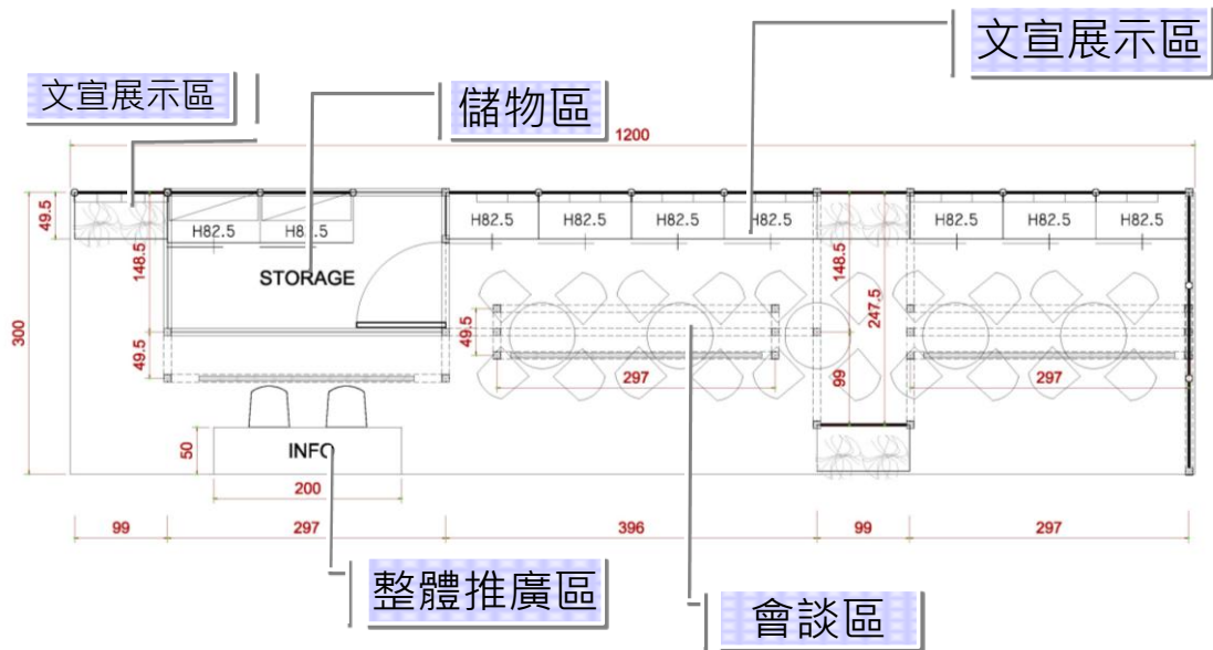
展場平面圖
