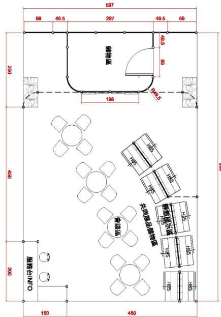
《臺灣攤位平面配置圖》
